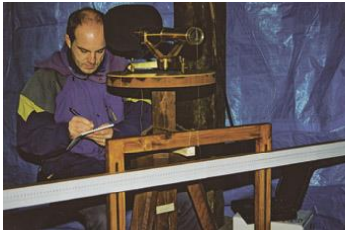
Beobachtungsfernrohr von Utzschneider und Fraunhofer (ca. 1860)
