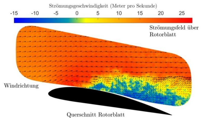
Abbildung 1: Mittels PIV gemessenen Strömungsabriss an einem Flügelprofil (Einzelaufnahme mit kolorierter Strömungsgeschwindigkeit)
