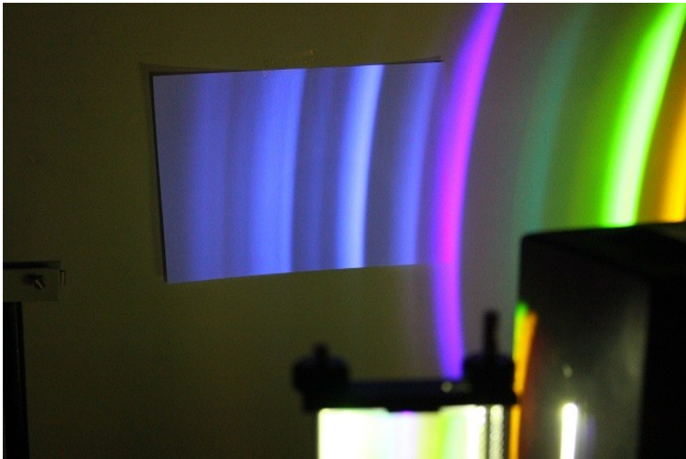
Abb. 10: Spektrum einer Quecksilberdampf Lampe ohne Glaskolben.
