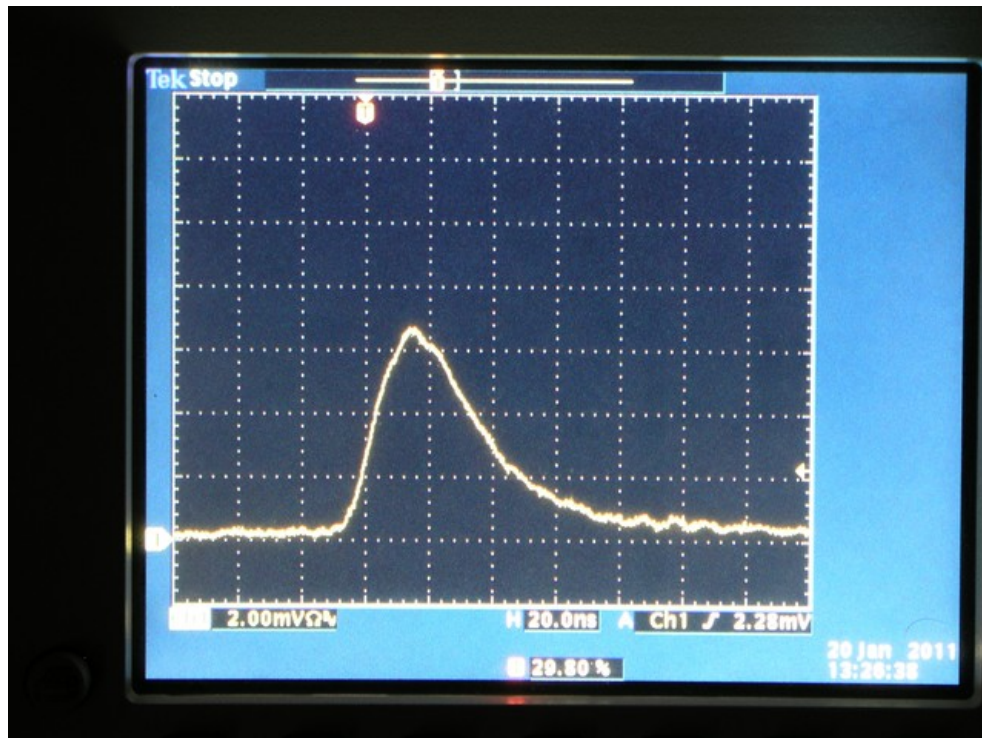
Abb. 4: Fluoreszenzsignal der Uranin-Probe, gemessen mit einer Photodiode.
