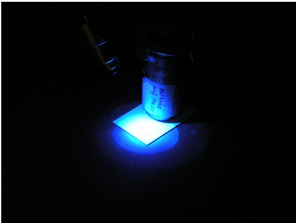
Abb. 9: Versuchsaufbau zur Phosphoreszenz. Das Plättchen wird mit Licht einer blauen LED angeregt und dann unter die Photozelle gezogen.
