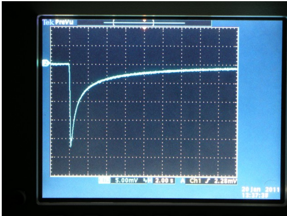
Abb. 8: Zeitlicher Verlauf der Phosphoreszenz des verwendeten Plättchens, gemessen mit einer Photozelle. Die Zeitkonstante liegt in der Größenordnung 1\text{ s} .
