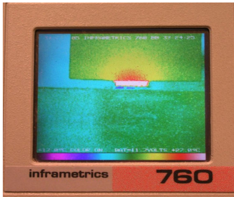
Abb. 2: Displaybild von einem Peltier-Element im Betrieb, Temperaturbereich: 17°C (Schwarz) bis 27°C (Weiß)
